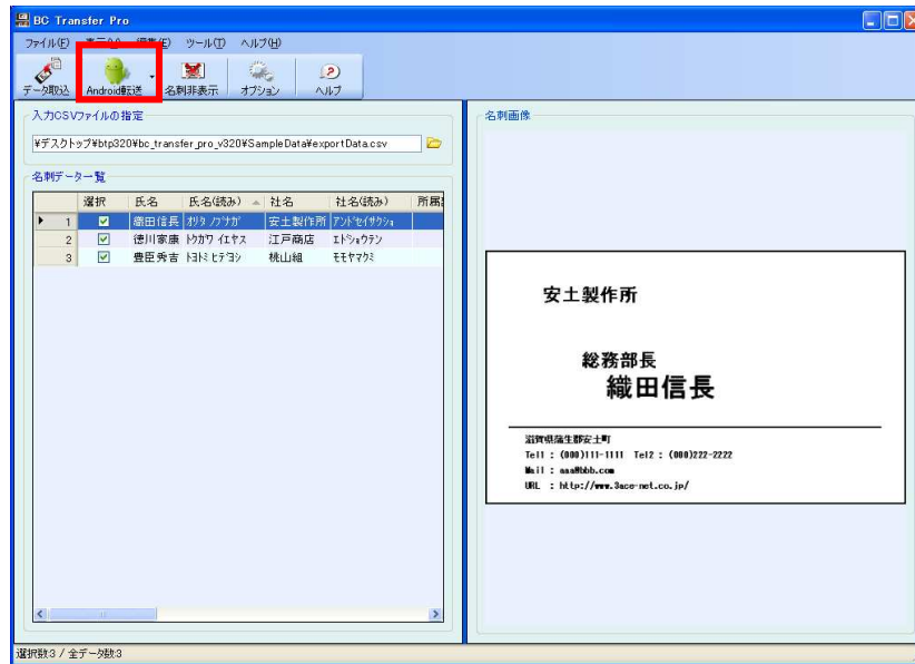
図 3 『BC Transfer Pro』メイン画面
